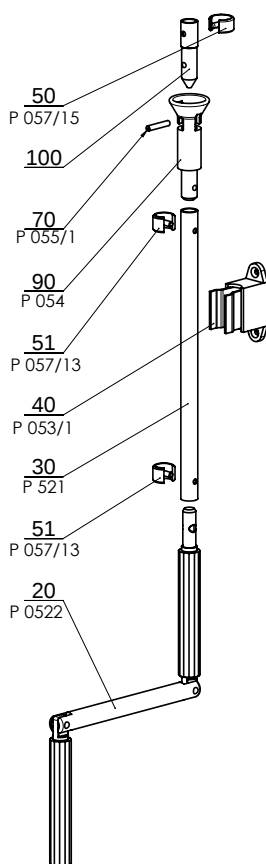
KLIKA ÚPLNÁ ODNÍMATELNÁ S PRŮCHODKOU 90° (pro SCREEN ZIP, LITE, GW)
