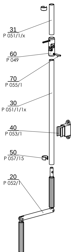
Klika úplná pro Screen ZIP (2-00868-XXXX-B)
